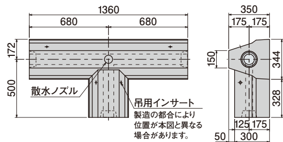
同心T型平L500
