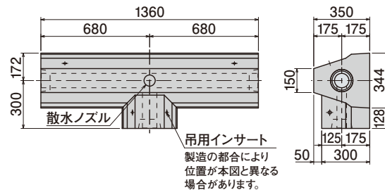
同心T型段L300
