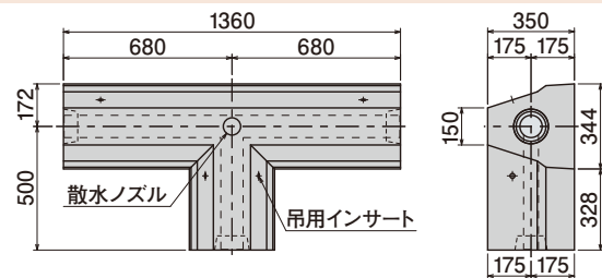
同心T型平L500
