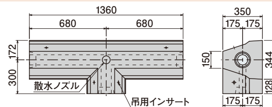
同心T型平L300
